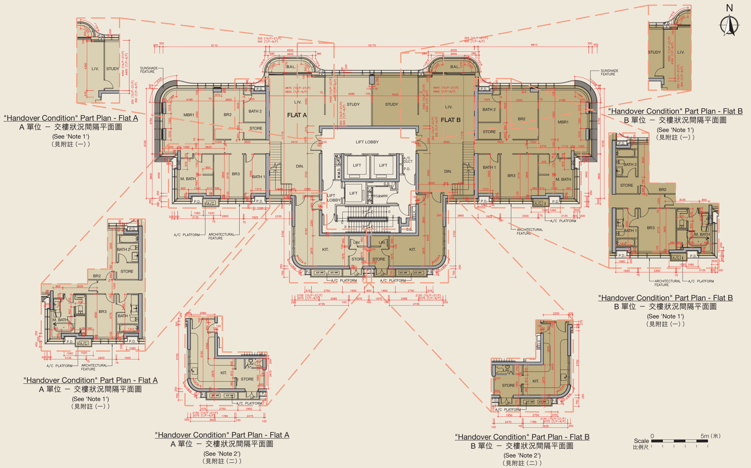
27/F Floor Plan 27 樓平面圖
